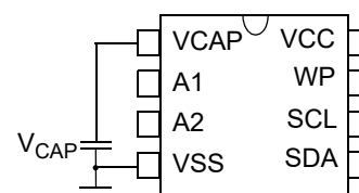
Fig. 10: PowerStore Cofiguration
